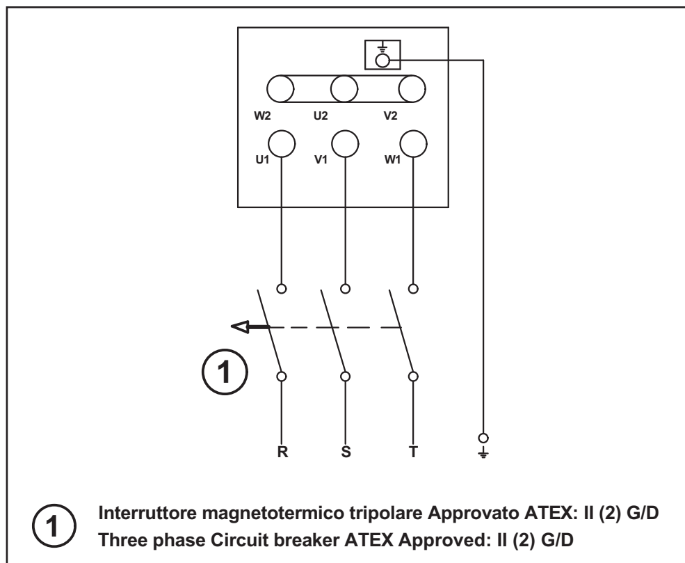
Shema vezave
